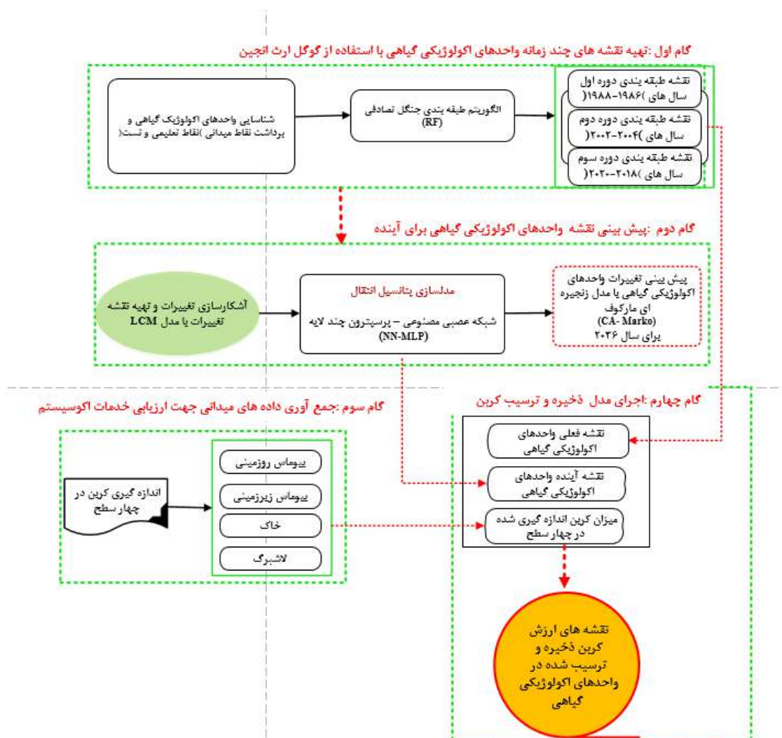
شکل ۳: مراحل برآورد خدمات اکوسیستم و تهیه نقشه های ذخیره و ترسیب کربن در واحدهای اکولوژیک گیاهی چهارگانه
