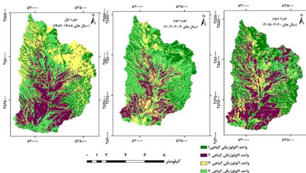
شکل ۴: نقشه طبقه‌بندی واحدهای اکولوژیک گیاهی با استفاده از الگوریتم طبقه‌بندی RF برای سه دوره اول، دوم و سوم
