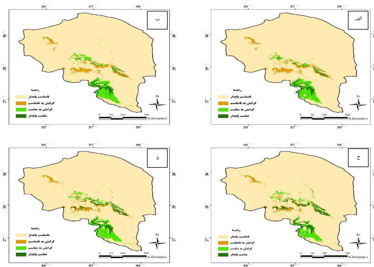
شکل ۴: تغییرات اندازه محدوده پراکنش گونه Tectrium polium تحت تأثیر تغییر اقلیم در سال ۲۰۵۰ در استان کرمان. الف) تغییرات اندازه محدوده پراکنش گونه تحت سناریو SSP245 مدل گردش عمومی HadGEM3-GC31-LL، ب) تغییرات اندازه محدوده پراکنش گونه تحت سناریو SSP585 مدل گردش عمومی HadGEM3-GC31-LL، ج) تغییرات اندازه محدوده پراکنش گونه تحت سناریو SSP245 مدل گردش عمومی MRI-ESM2-0، د) تغییرات اندازه محدوده پراکنش گونه تحت سناریو SSP585 مدل گردش عمومی MRI-ESM2-0.
