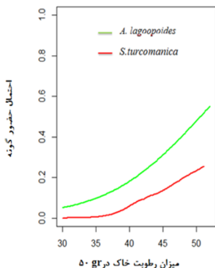
شکل (۱) برازش تابع HOF به درصد رطوبت
