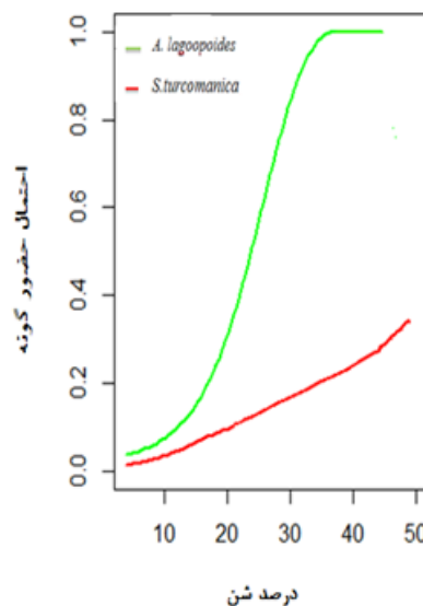
شکل (۲) برازش تابع HOF به درصد شن
