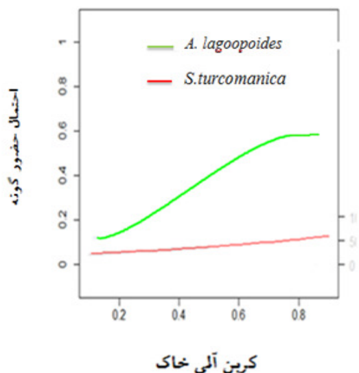
شکل (۹) برازش تابع HOF به وزن Ec خاک شکل (۱۰) برازش تابع HOF به کربن آلی خاک
