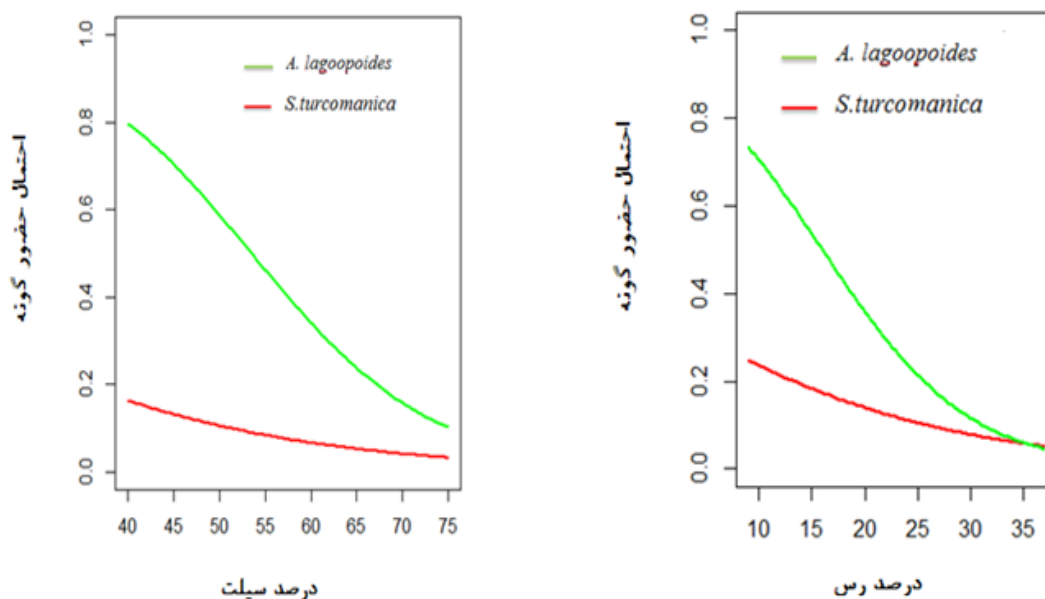
شکل (۳) برازش تابع HOF به درصد سیلت شکل (۴) برازش تابع HOF به درصد رس
