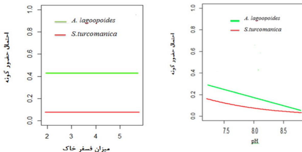
شکل (۵) برازش تابع HOF به میزان فسفر خاک شکل (۶) برازش تابع HOF به اسیدیته خاک
