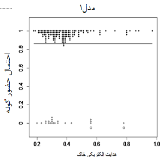
شکل ۶: برازش تابع HOF به متغیر هدایت الکتریکی
