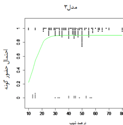
شکل ۵: برازش تابع HOF به متغیر شیب دامنه
