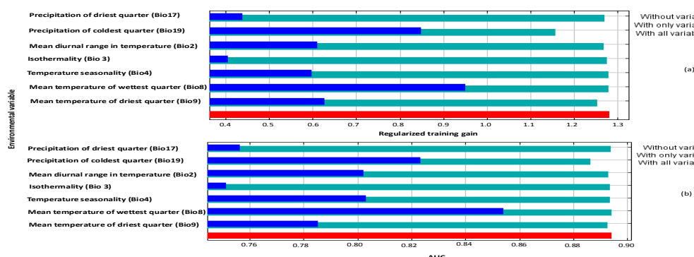
شکل ۲- قدرت تخمین نسبی اثرات متغیرهای زیست اقلیمی متفاوت به دست آمده از Jackknife در مدل مکسنت (a) قدرت پیشگویی در مدل کالیبراسیون و (b) AUC، سطح زیر منحنی در مدل تست. مقادیر از متوسط ۱۰ بار اجرای مدل به دست آمده‌اند.
