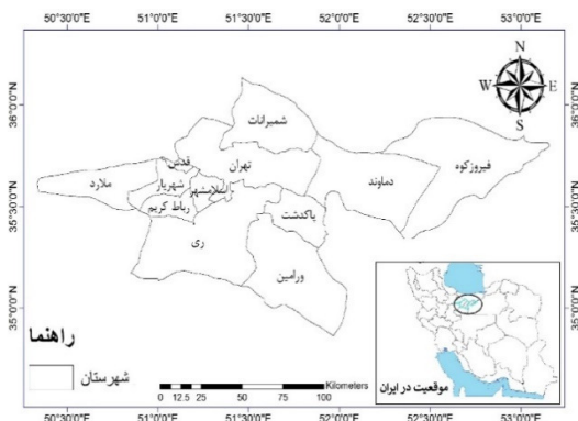
شکل ۱: موقعیت استان تهران و شهرستان های آن
