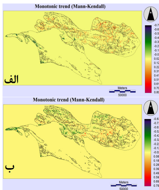
شکل ۷: نقشه مناطق دارای روند معنی‌دار شروع فصل رشد
