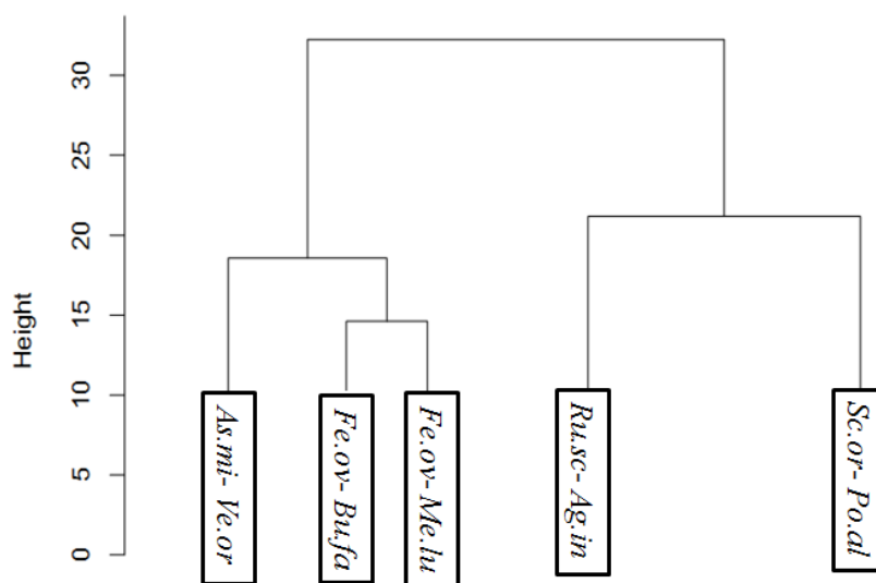
شکل ۲: دیاگرام طبقه‌بندی پوشش گیاهی در محدوده معدن مس سونگون (هر زیراجتماع بر اساس دو گونه غالب مشخص شده است) ( Me.lu )، Bupleurum falcatum ( Bu.fa )، Festuca ovina ( Fe.ov )، Verbascum oreophilum ( Ve.or )، Astragalus microcephalus ( As.mi ) ( Polygonum alpestre ( Po.al )، Scariola orientalis ( Sc.or )، Agropyron intermedium ( Ag.in )، Rumex scutatus ( Ru.sc )، Medicago lupulina ).
