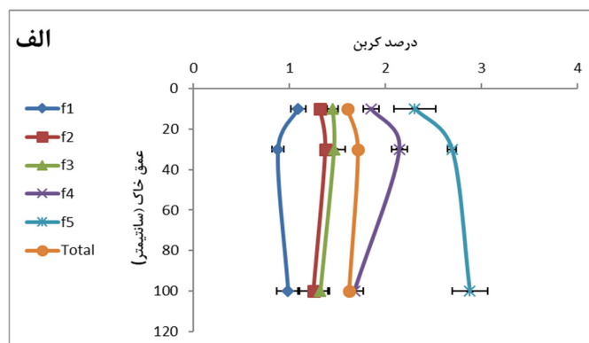
شکل ۳: نمودار توزیع کربن ( \pm اشتباه معیار) در اجزاء اندازه‌ای خاک در اعماق مختلف پارک ملی (F1: 1000- 2000 \mu m).
