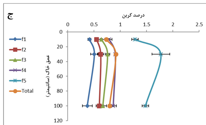
شکل ۵: نمودار توزیع کربن ( \pm اشتباه معیار) در اجزاء اندازه‌ای خاک در اعماق مختلف منطقه شکار ممنوع (F1: 1000- 2000 \mu m).
