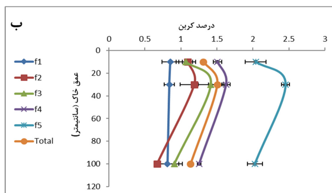
شکل ۴: نمودار توزیع کربن ( \pm اشتباه معیار) در اجزاء اندازه‌ای خاک در اعماق مختلف منطقه حفاظت‌شده (F1: 1000- 2000 \mu m).
