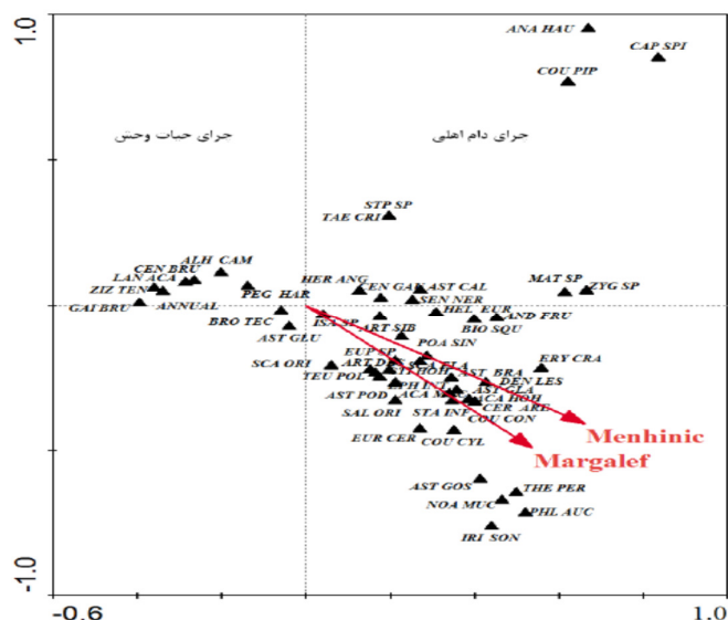
شکل ۳: نمودار سه پلاتی گونه- مکان - محیط حاصل از رجبندی CCA ( اسامی کامل گونه‌ها در جدول ۲ آمده است).
