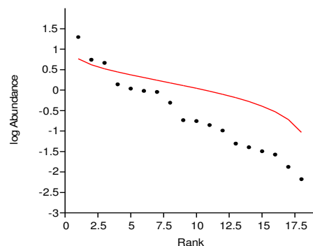
شکل ۲- نمودار عصای شکسته در منطقه تحت چرای دام اهلی (الف) و منطقه تحت چرای حیات وحش (ب).
