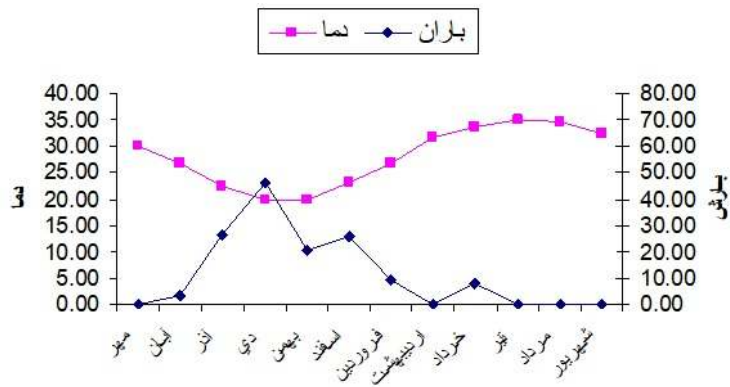
شکل ۲: منحنی آمپروترمیک منطقه مورد مطالعه در یک دوره آماری ۳۰ ساله
