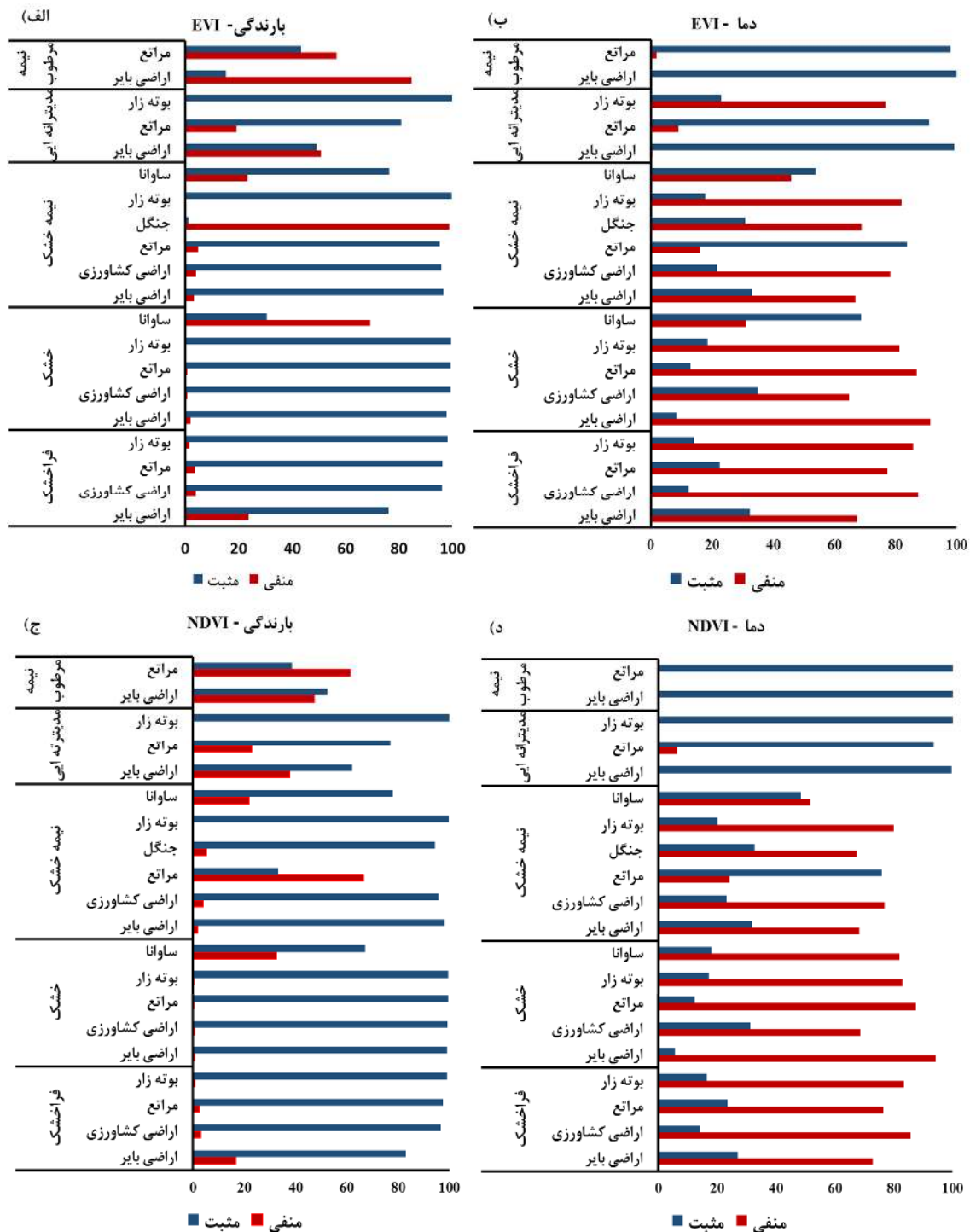
شکل ۱۱: همبستگی بین EVI و بارندگی (الف)، EVI و دما (ب)، NDVI و بارندگی (ج)، و NDVI و دما (د) در کاربری‌های مختلف در بازه زمانی سال ۲۰۰۱-۲۰۲۰
