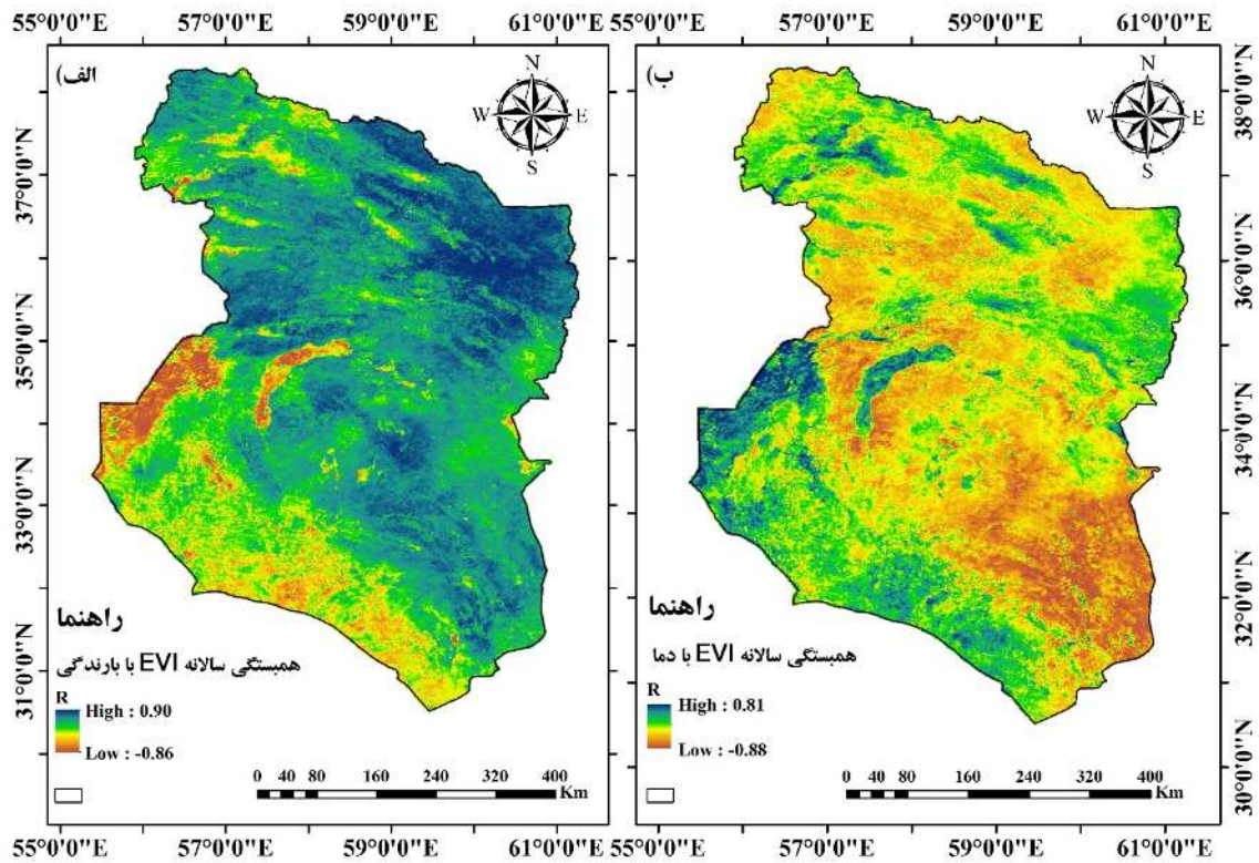
شکل ۸: الف) همبستگی بین EVI و بارندگی، ب) همبستگی EVI و دما در بازه زمانی سال ۲۰۰۱-۲۰۲۰
