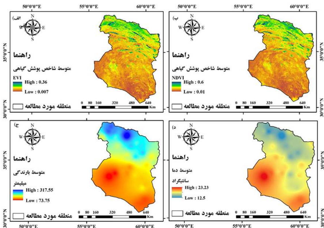
شکل ۶: میانگین ۲۰ ساله (الف) EVI، (ب) NDVI، (ج) بارندگی، (د) دما در بازه زمانی ۲۰۰۱-۲۰۲۰
