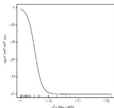
شکل ۱۵: منحنی پاسخ شاخص سطح برگ - روش خطی تعمیم‌یافته
