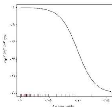
شکل ۲۴: منحنی پاسخ شاخص سطح برگی - روش رگرسیون تطبیقی چند متغیره اسپیلاین
