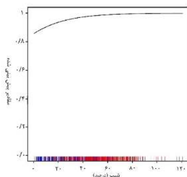
شکل ۱۱: Error! No text of specified style in document. منحنی پاسخ شیب - روش خطی تعمیم‌یافته
