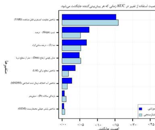
شکل ۸: نمودار اهمیت هر یک از متغیرها بر مدل مطلوبیت زیستگاه J. excelsa در روش خطی تعمیم‌یافته
