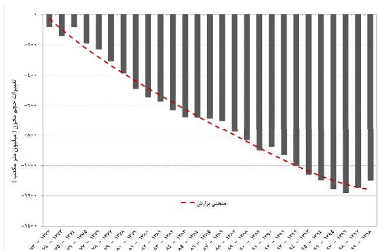
شکل ۵: نمودار تغییرات تجمعی حجم مخزن آبخوان آبرفتی برای دوره (۱۳۸۰-۱۳۹۹) آبخوان‌های گرمسار، فیروزکوه، دماوند و همد-آب‌سرد
