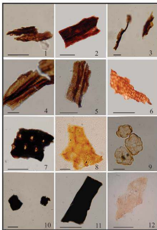
Figs. 1- 8: Plant tissues; Fig ۹- پلیت ۳. شکل ۱۰- پلیت ۳ 9: Algal spores; Fig 10: Equidimensional Opaque palynomacer; Fig 11: Blade-shape Opaque palynomacer; Fig 12: Transparent AOM. Scale bar equals 20 μm
