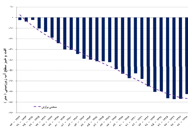
شکل ۴: نمودار تغییرات تجمعی سطح آب زیرزمینی برای یک دوره ۱۹ ساله (۱۳۸۰-۱۳۹۹) آبخوان‌های گرمسار، فیروزکوه، دماوند و همد-آبسرده
