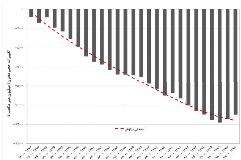
شکل ۵: نمودار تغییرات تجمعی حجم مخزن آبخوان آبرفتی برای دوره (۱۳۸۰-۱۳۹۹) آبخوان‌های گرمسار، فیروزکوه، دماوند و همد-آبسر
