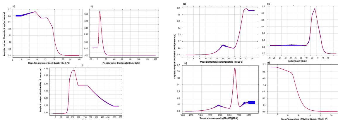
شکل ۳- نمودار پاسخ رابطه بین احتمال حضور گونه D. mucronata با هفت متغیر اقلیمی تاثیر گذار بر پراکنش آنرا نشان می‌دهد. (a) متوسط دامنه درجه حرارت روزانه (Bio 2; °C)، (b) همدامی (Bio 3)، (c) درجه حرارت فصلی (Bio 4)، (d) متوسط درجه حرارت مرطوب‌ترین سه ماه پیوسته سال (Bio 8; °C)، (e) متوسط درجه حرارت خشک‌ترین سه ماه پیوسته سال (Bio 9; °C)، (f) مقدار بارندگی در خشک‌ترین سه ماه پیوسته سال (Bio 17; mm)، (g) مقدار بارندگی در مرطوب‌ترین سه ماه پیوسته سال (Bio 19; mm) (برای اطلاعات در مورد نحوه محاسبه این متغیرها به منبع ۳۰ مراجعه شود)
