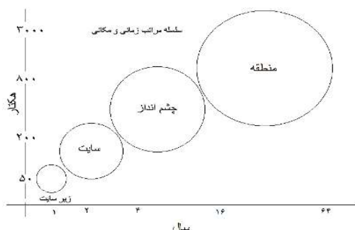
شکل ۴- سلسله مراتب مکانی و زمانی منظور شده جهت آنالیز داده‌ها (طراحی توسط محقق با توجه به طرح آزمایش و اهداف تحقیق)
