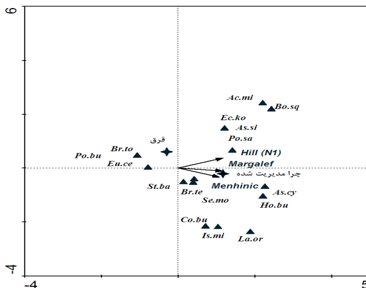
شکل ۵- نمودار سه پلاتی گونه-مکان-محیط حاصل از رج‌بندی CCA (اسامی کامل گونه‌های گیاهی در جدول ۴ آورده شده است)
