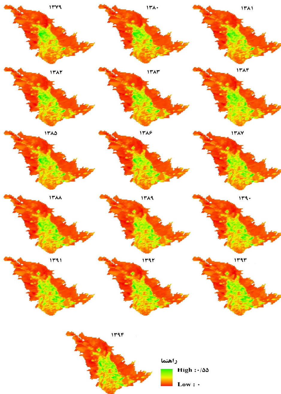
شکل ۶: پهنه‌بندی شاخص پوشش گیاهی NDVI در بازه زمانی ۲۰۱۵-۲۰۲۰
