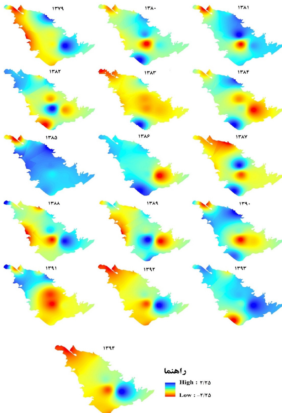
شکل ۳: پهنه‌بندی شاخص خشکسالی SPI در بازه زمانی ۲۰۰۰-۲۰۱۵
