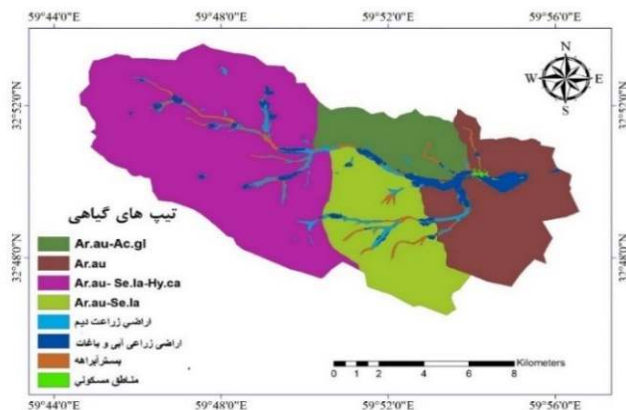
شکل ۲: تیپ‌های گیاهی مراتع کوهستانی در میان
