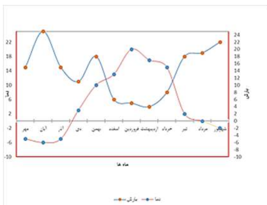
شکل ۱: منحنی آمبروترمیک
