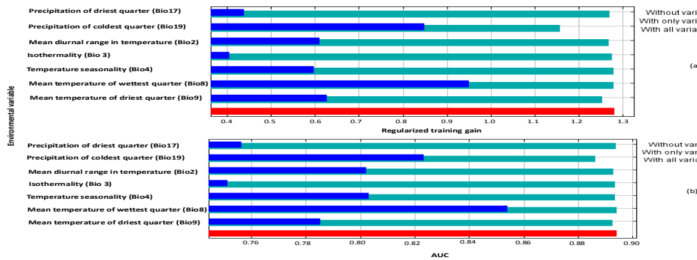
شکل ۲- قدرت تخمین نسبی اثرات متغیرهای زیست اقلیمی متفاوت به دست آمده از Jackknife در مدل مکسنت (a) قدرت پیشگویی در مدل کالیبراسیون و (b) AUC، سطح زیر منحنی در مدل تست. مقادارها از متوسط ۱۰ بار اجرای مدل به دست آمده‌اند.
