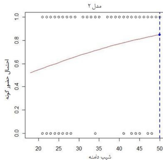
شکل ۶: برازش تابع HOF به متغیر شیب دامنه
