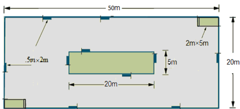
شکل ۲- پلات ویتاگر تعدیل شده (۲۴)
