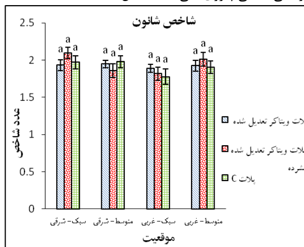
شکل ۸- مقایسه شاخص شانون وینر در پلات‌های مختلف
