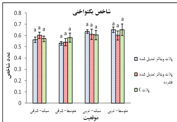
شکل ۷- مقایسه شاخص یکنواختی در پلات‌های مختلف
