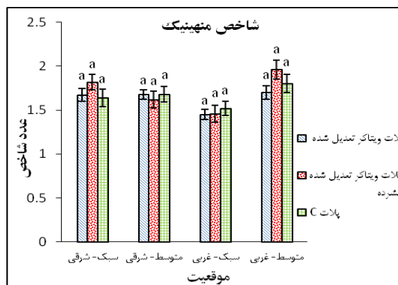
شکل ۵- مقایسه شاخص منهنیک در پلات‌های مختلف
