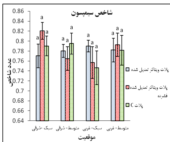
شکل ۹- مقایسه شاخص سیمپسون در پلات‌های مختلف
