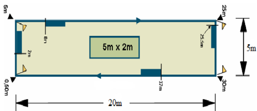
شکل ۳- پلات ویتاگر تعدیل شده فشرده (۳)
