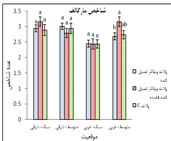
شکل ۶- مقایسه شاخص مارگالف در پلات‌های مختلف
