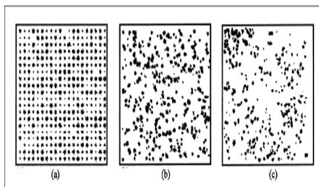
شکل ۵: سه نوع الگوی پراکنش گیاهی شامل (a) یکنواخت (b) تصادفی و (c) کپهای (برگرفته از لودیگ و رینولد، ۱۹۷۵).
