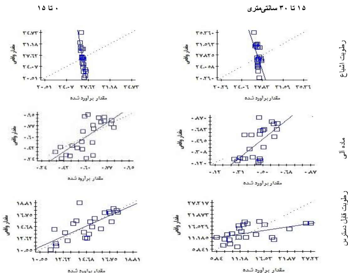
شکل ۳- مقایسه بین مقادیر اندازه گیری (محور عمودی) و برآورد شده (محور افقی) رطوبت اشباع (ساختر مکانی ضعیف)، ماده آلی (ساختر مکانی متوسط) و رطوبت قابل دسترس (ساختر مکانی قوی) در دو عمق مورد بررسی
