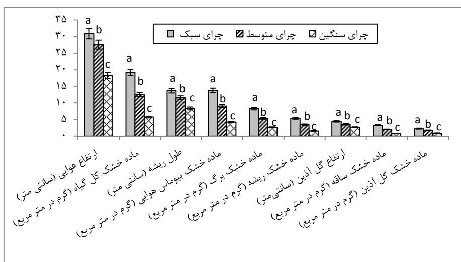
شکل ۱- گروه بندی میانگین اندام های گیاهی شدت های مختلف چرای در دامنه های مورد مطالعه میانگین هر شاخص با حرف غیر مشترک (a, b, c) بیانگر وجود اختلاف معنی دار می باشد
