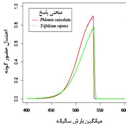
شکل ۱۲- برازش تابع HOF به متغیر بارش
