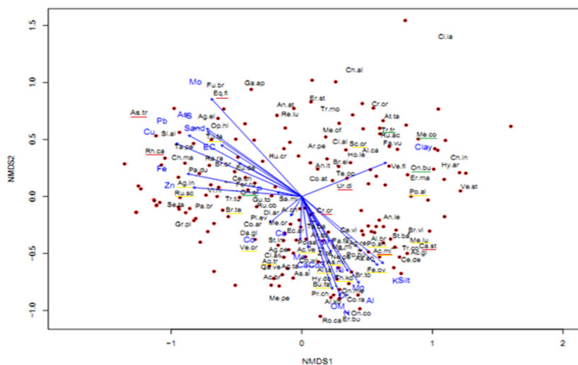
شکل ۴: تجزیه و تحلیل NMDS به منظور بررسی ارتباط گونه‌های گیاهی با خصوصیات خاک در محدوده معدن مس سونگون مخفف نام گونه‌های گیاهی از دو حرف اول نام جنس و دو حرف اول نام گونه است که مهمترین گونه‌ها عبارتند از:
