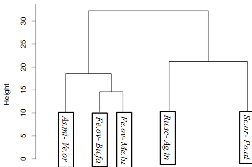
شکل ۲: دیاگرام طبقه‌بندی پوشش گیاهی در محدوده معدن مس سونگون (هر زیراجتماع بر اساس دو گونه غالب مشخص شده است) (Me.lu) Bupleurum falcatum (Bu.fa) Festuca ovina (Fe.ov)، Verbascum oreophilum (Ve.or) Astragalus microcephalus (As.mi) ( Polygonum alpestre (Po.al) Scariola orientalis (Sc.or) Agropyron intermedium (Ag.in) Rumex scutatus (Ru.sc) Medicago lupulina
