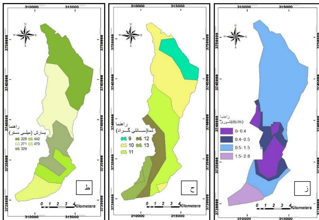
شکل ۳: نقشه‌های وکتوری حوزه آبخیز هیراب (الف) شیب، (ب) ارتفاع، (ج) جهت، (د) بافت خاک، (ه) عمق خاک، (و) اسیدبته، (ز) شوری خاک، (ح) دما و (ط) بارش
