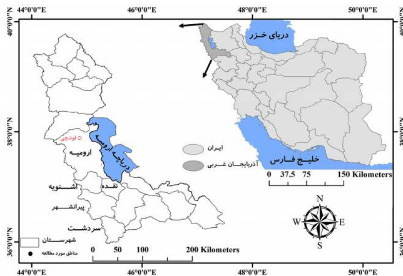
شکل ۱: موقعیت مکانی سایت قوشچی در استان آذربایجان غربی و در ایران
