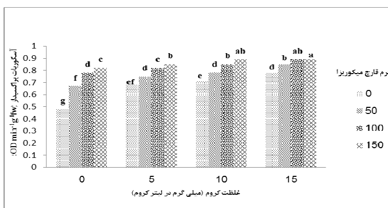
شکل ۸- اثر متقابل کروم*میکوریزا بر میانگین فعالیت آنزیم آسکوربات پراکسیداز در سورگوم
