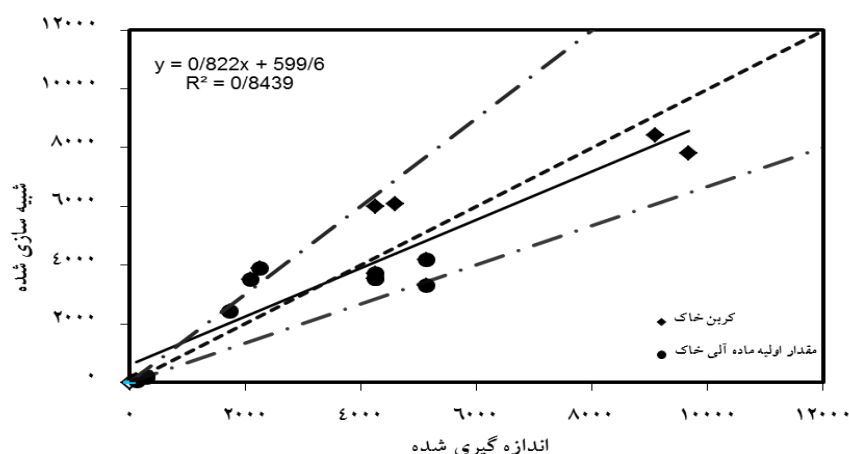
شکل ۲- مؤلفه‌های خاکی شبیه‌سازی شده توسط مدل CENTURY در مقابل مقادیر اندازه‌گیری شده آن‌ها، خط پر معادله رگرسیون، خط چین وسط، خط ۱:۱ و خطوط نقطه چین، حدود اطمینان خط رگرسیون هستند.
