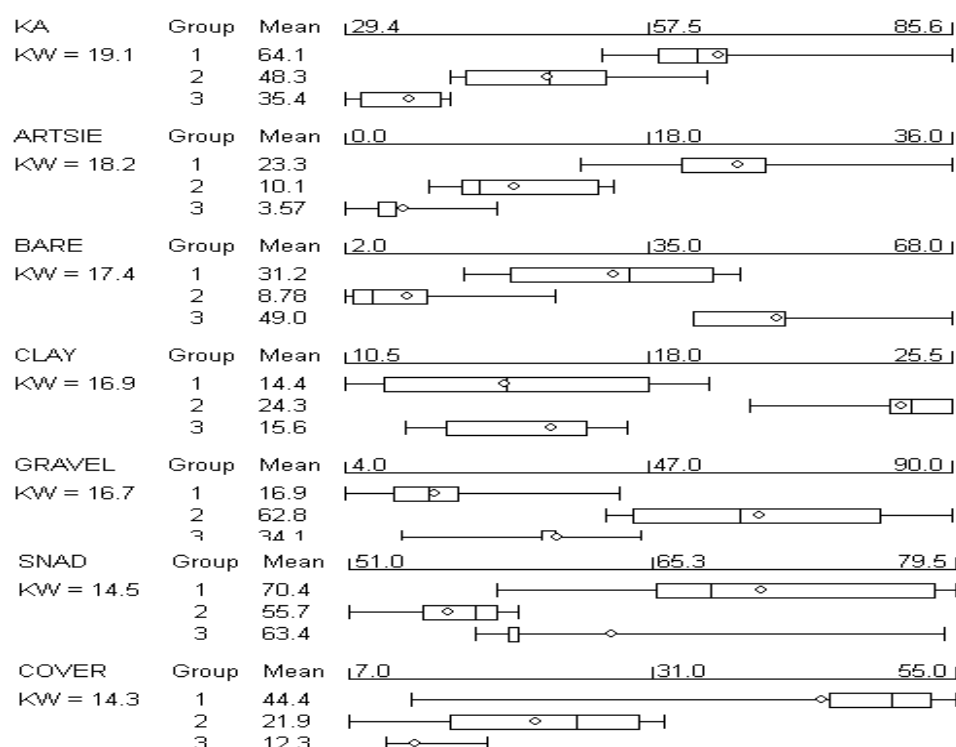
شکل ۲- نمودار Box-Whisker (ارزیابی با آنالیز ANOSIM و آنالیز کروسکال والیز انجام شد). بالاترین مقادیر کروسکال والیز برای متغیرهای پتاسیم سطحی خاک (KA)، درصد تاج پوشش درمنه دشتی (ARTSIE)، خاک لخت (BARE)، رس (CLAY)، سنگ و سنگریزه (GRAVEL)، شن (SAND) و میزان درصد تاج پوشش کل گونه ها (COVER) مشاهده گردید و این عوامل در تفکیک گروه ها در دندوگرام بیشترین تاثیر را داشته‌اند.
