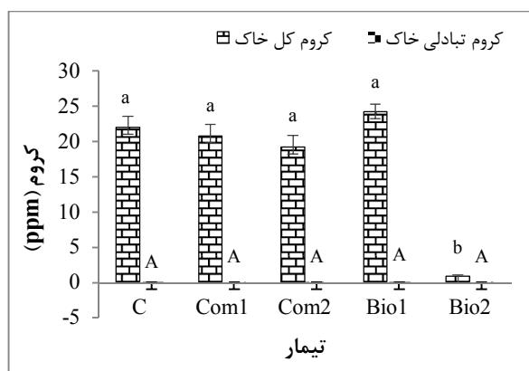
شکل ۸- تأثیر تیمارها بر غلظت کروم کل و تبدیلی خاک
