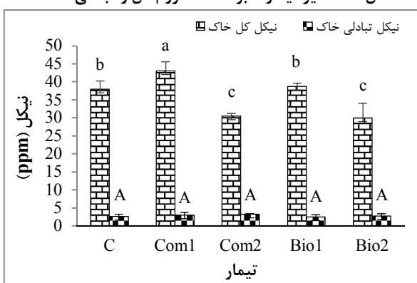
شکل ۱۰- تأثیر تیمارها بر غلظت نیکل کل و تبدیلی خاک
